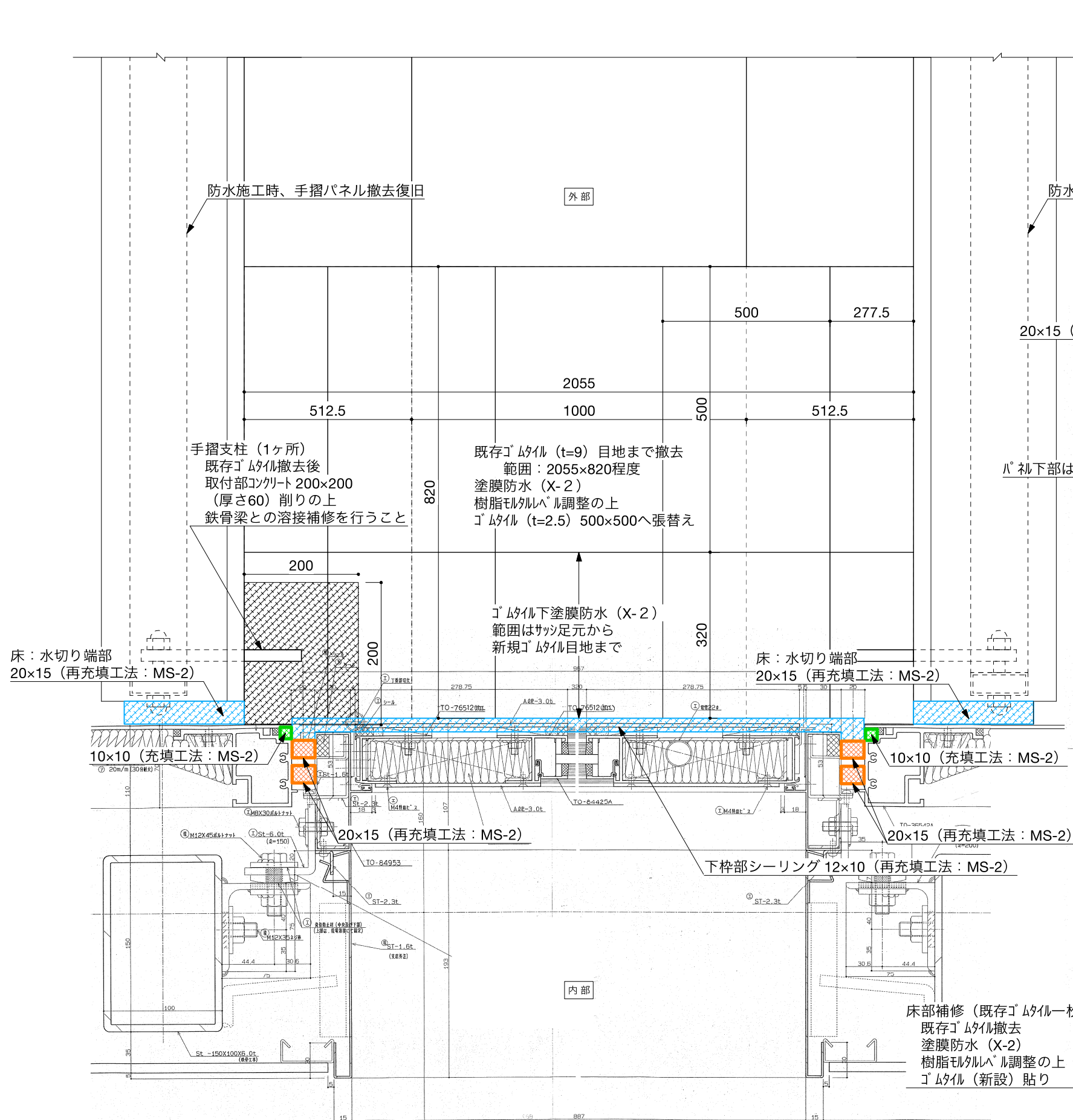
矢視部 1 4 平面詳細図 (3階片開き扉部)
