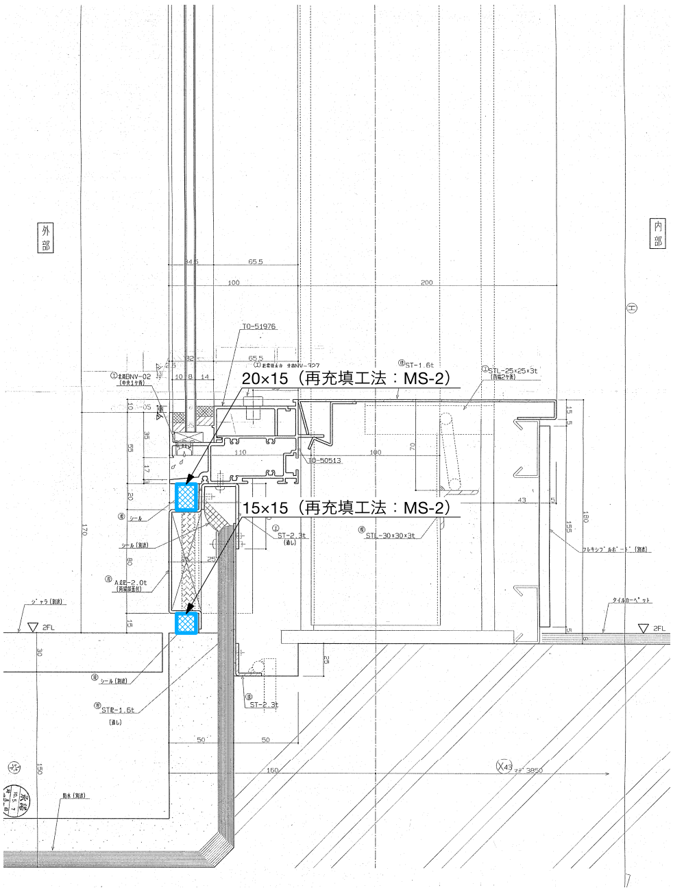
矢視部 5 断面詳細図 (2階サッシ部足元)
