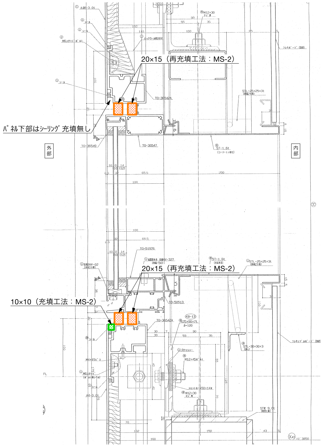
矢視部 2 断面詳細図 (一般部)
