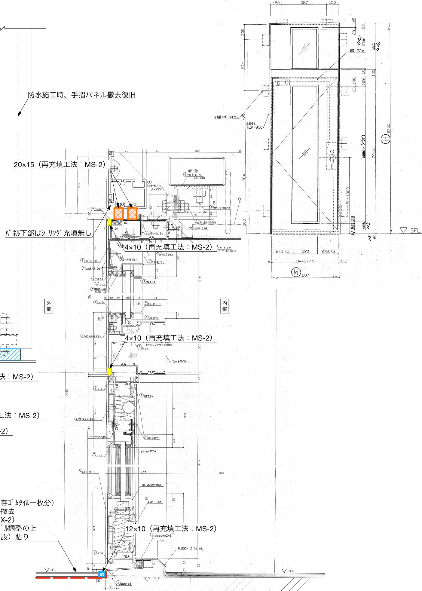
矢視部 1 5 断面詳細図 (3階片開き扉部)
