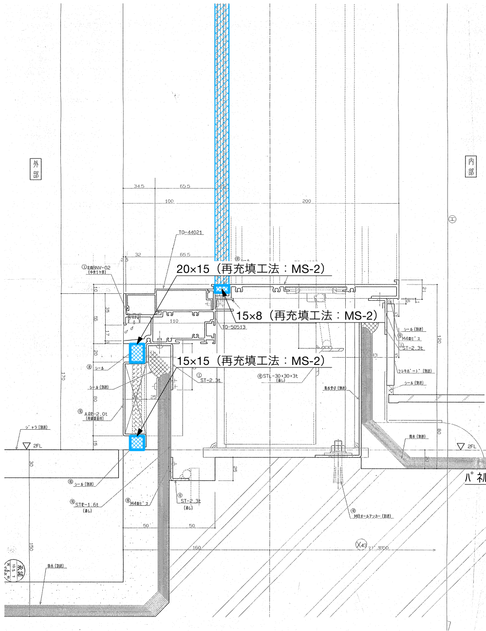
矢視部 3 断面詳細図 (2階開口部足元)
