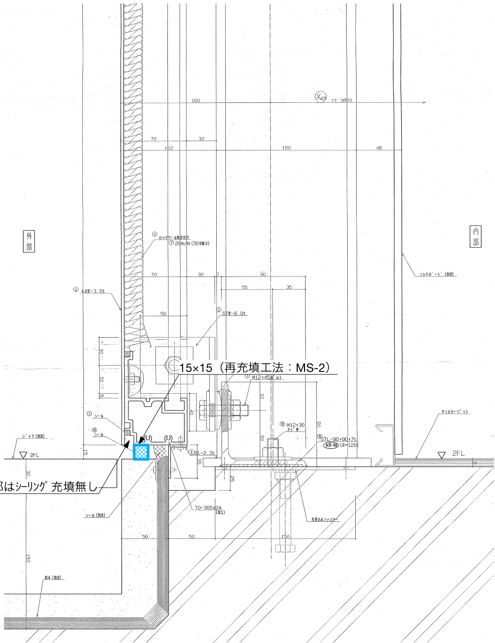
矢視部 4 断面詳細図 (2階ハコ部足元)
