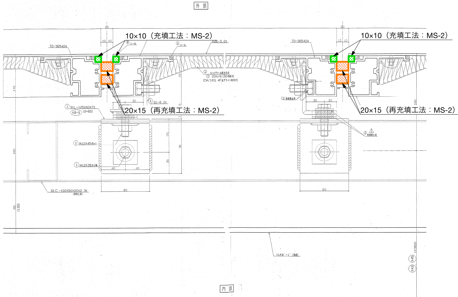
矢視部 1 3 平面詳細図 (パネル間取合い部)
