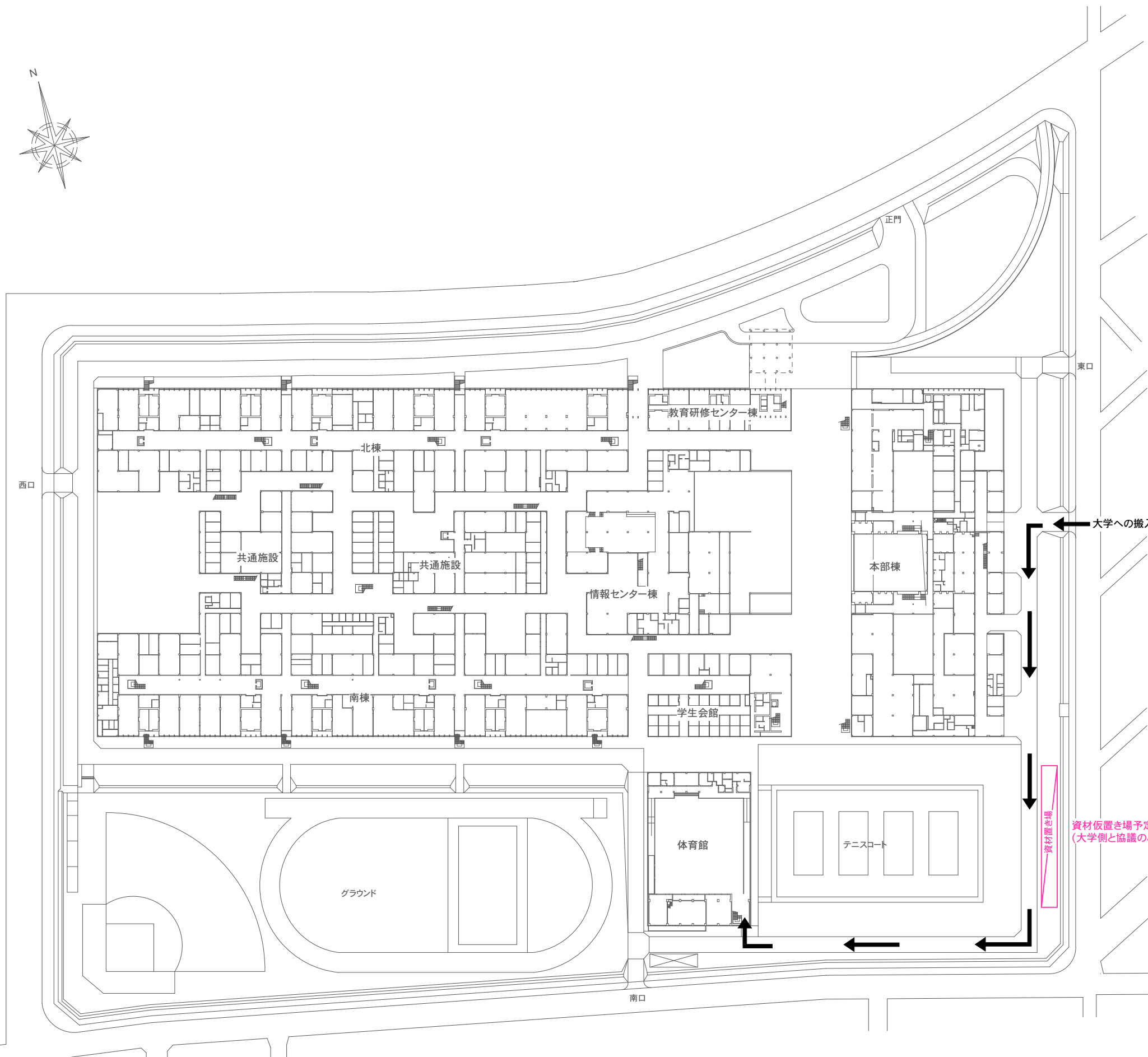
配置図 S=1/800
